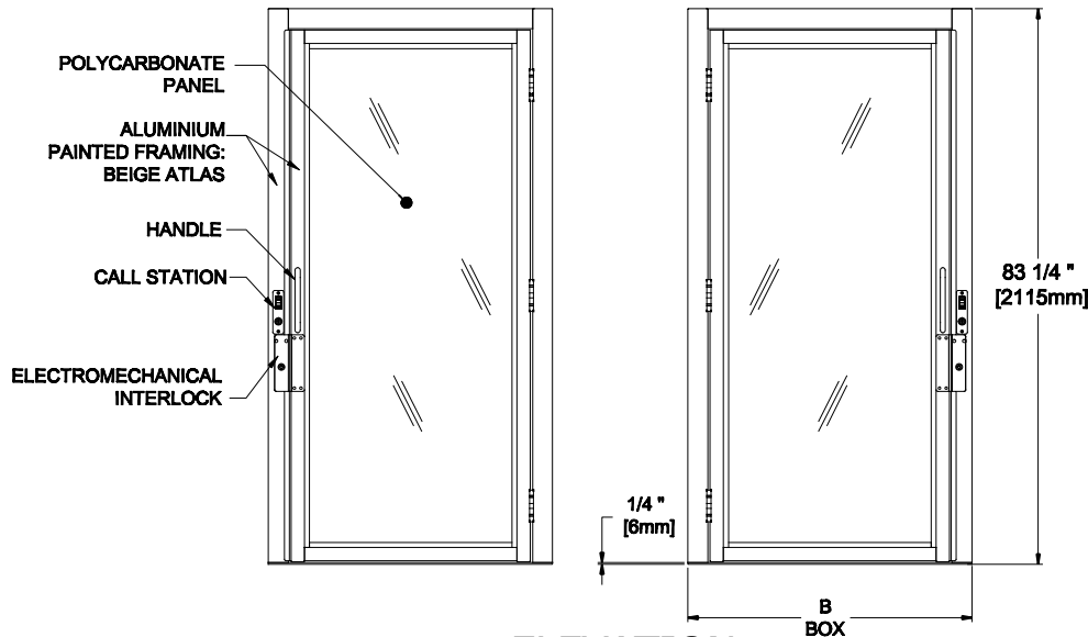
ELEVATION
